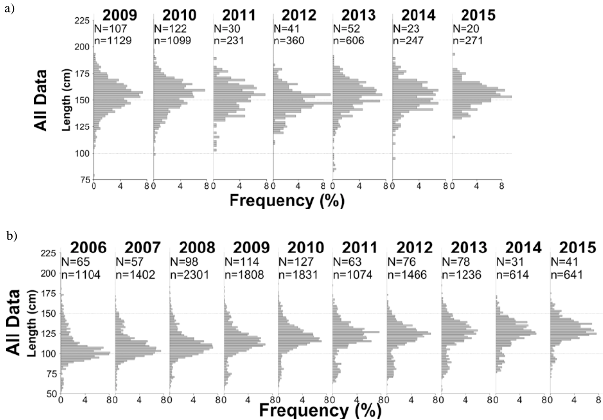
Figure 1 : Distributions des fréquences annuelles de longueur de : a) Dissostichus mawsoni , et b) D. eleginoides dans la sous-zone 48.4. Le nombre de poses desquelles des poissons ont été mesurés (N) et le nombre de poissons mesurés (n) par année sont précisés.
