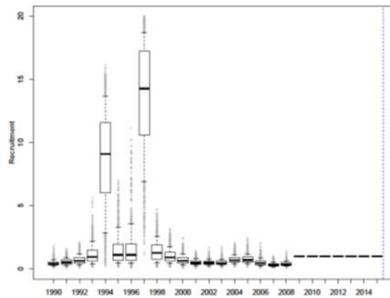
Figure A3 : Dissostichus eleginoides dans la sous-zone 48.4 : Recrutement estimé par MCMC avec abondance fixe des classes d'âges de 2009 à 2015.
