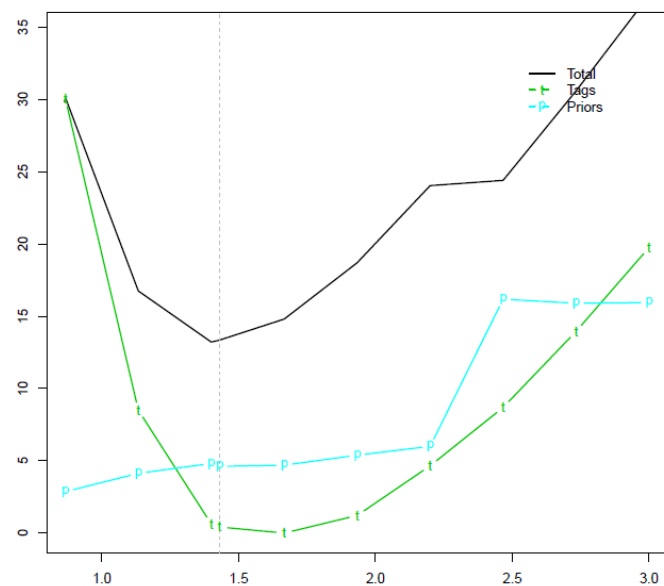
Figure A1 : Dissostichus eleginoides dans la sous-zone 48.4 : Profils de vraisemblance de valeurs de B_0 . Les valeurs de la log-vraisemblance négative ont été remises à l'échelle pour avoir un minimum de 0 pour chaque jeu de données. La ligne verticale indique l'estimation générale de la MPD de B_0 .
