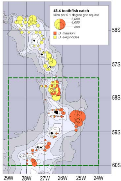
Figure 2 : Répartition des captures des deux espèces de Dissostichus dans la sous-zone 48.4.
