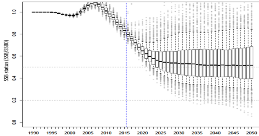
Figure A2 : Dissostichus eleginoides dans la sous-zone 48.4 : État de la biomasse du stock reproducteur estimé sur une période de projection de 35 ans pour un rendement constant de 47 tonnes. Les boîtes indiquent les 25 e et 75 e centiles. Les « moustaches » s'étendent jusqu'aux 5 e et 95 e centiles.
