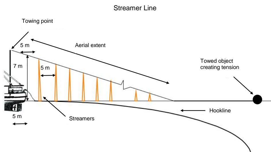
Figure 1 : Exemple des mesures de hauteur et d'espacement d'une ligne de banderoles.
